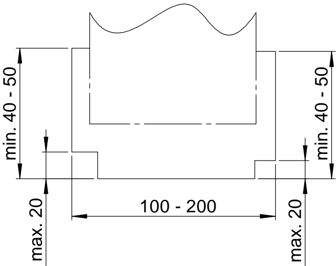
Masse der Türzarge (Masse eintragen und zurücksenden)
