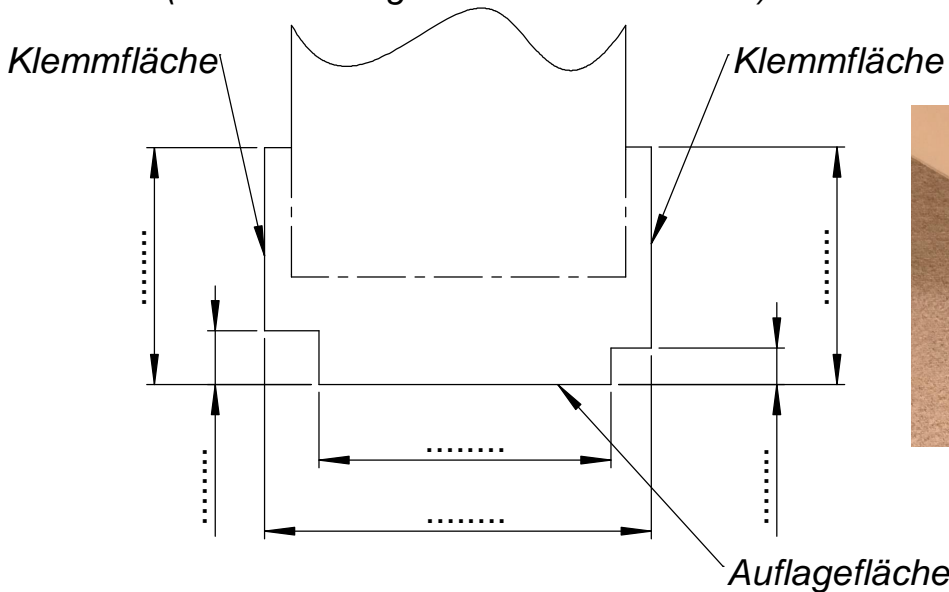
Masse der Türzarge (Masse eintragen und zurücksenden)
